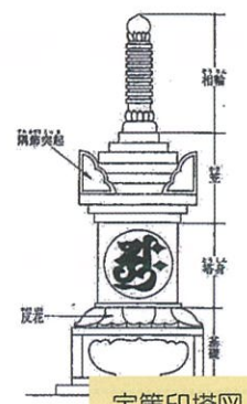
宝篋印塔図
