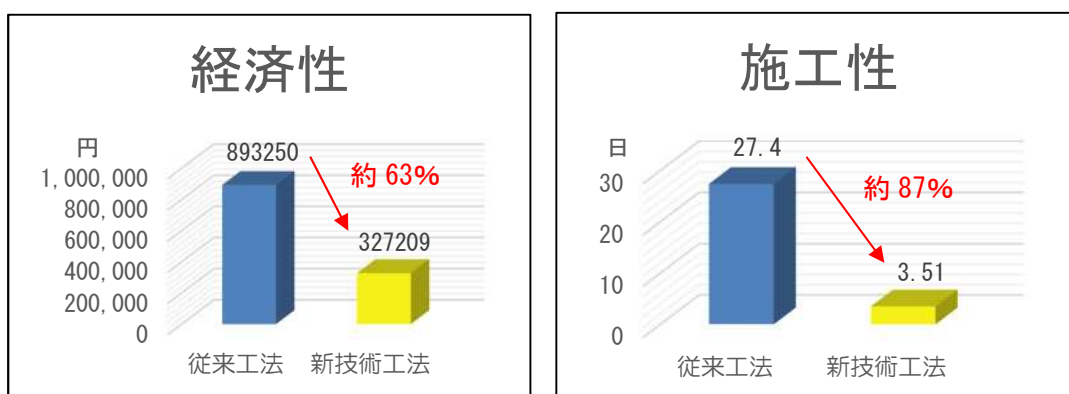
トンネル壁面の剥離防止工（はつり落とし+断面修復）15㎡当たりの比較
