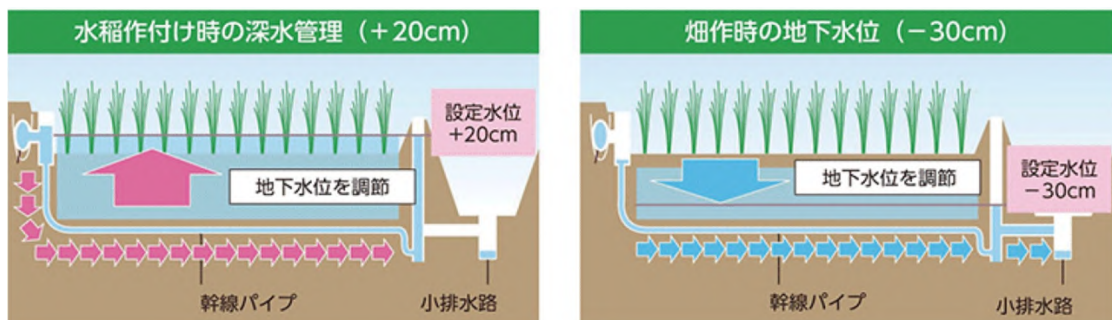
地下水位制御システムFOEASの概要
