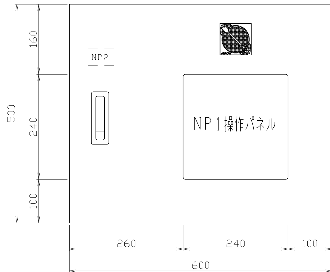
正面図
