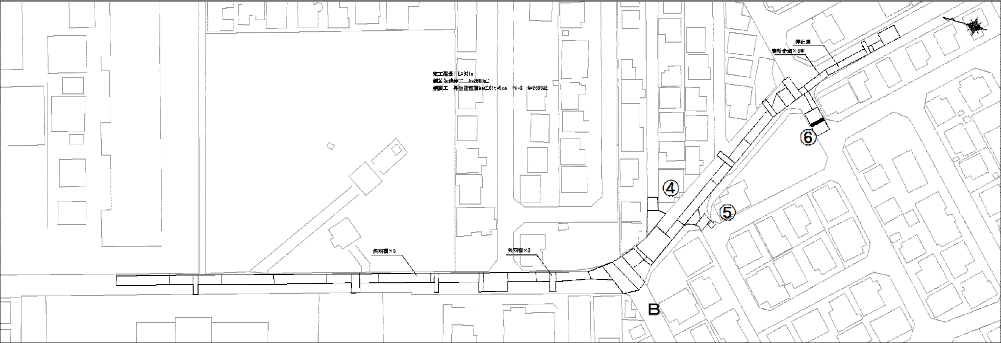
市道最上街道線平面図 S=1 : 100
