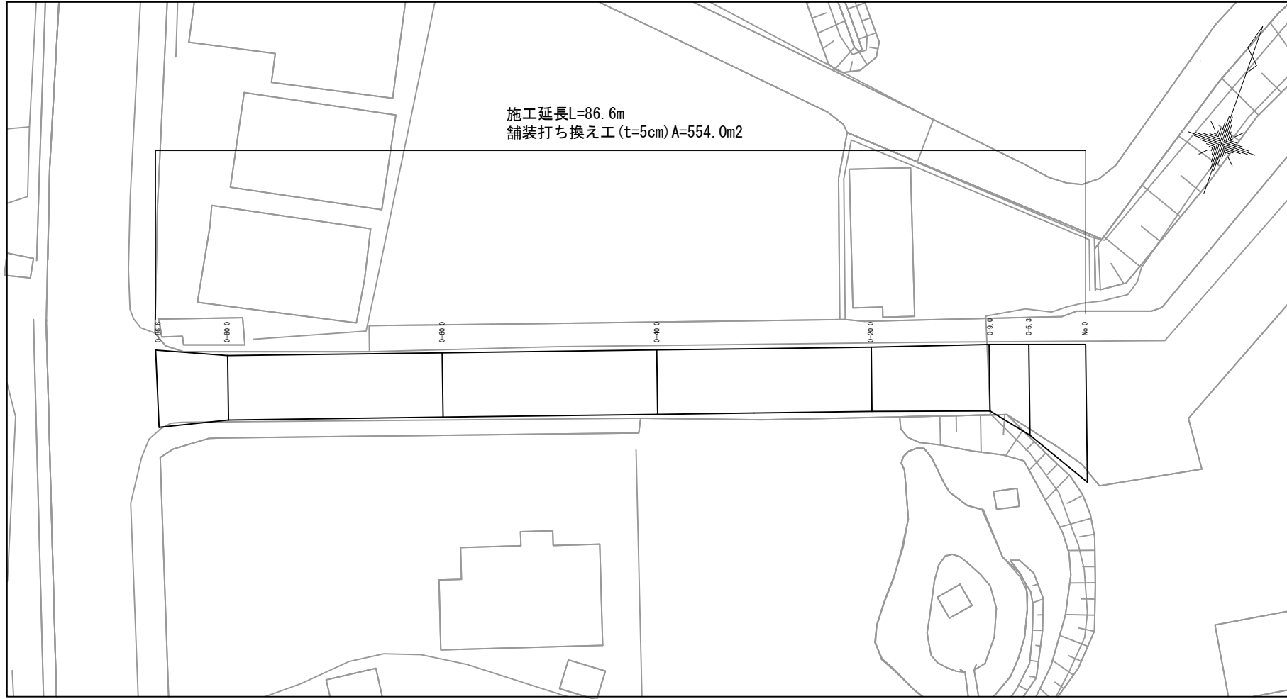
平面図 S=1:500
