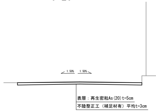
標準断面図 S=1:50
