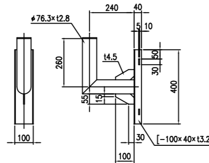
⑧ 電柱取付金具詳細図 S=1/20
