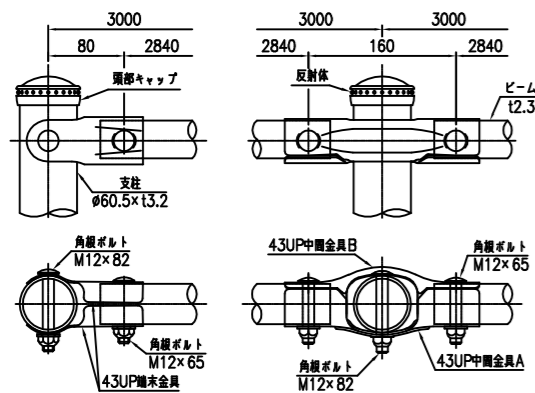
取付部詳細図 S=1:8
