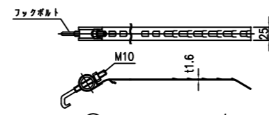
⑨ 取付バンド詳細図 S=1/10
