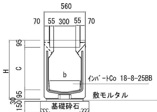
寸法表
