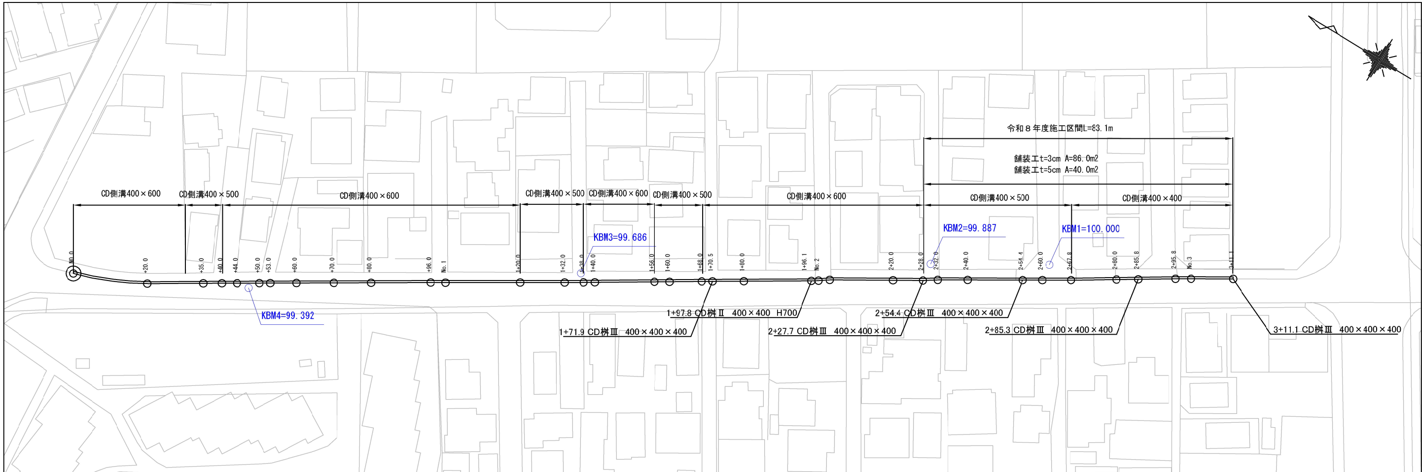
平面図 S=1:1000
