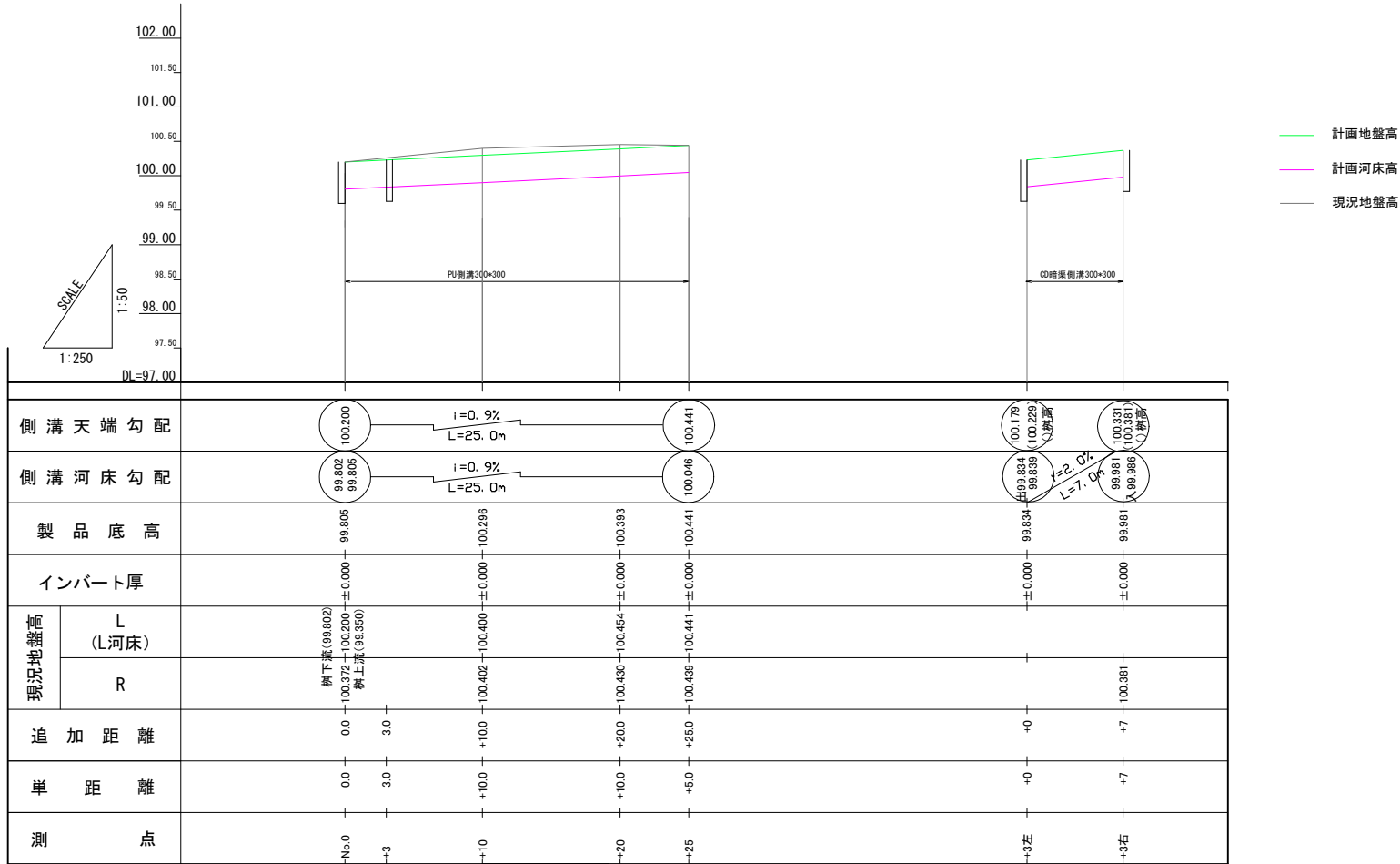
縦断面図 H=1:250 V=1:50
