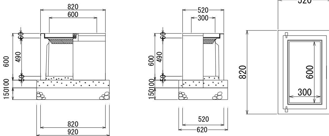
PU-3用柵300×600×H600 1基当たり材料表
