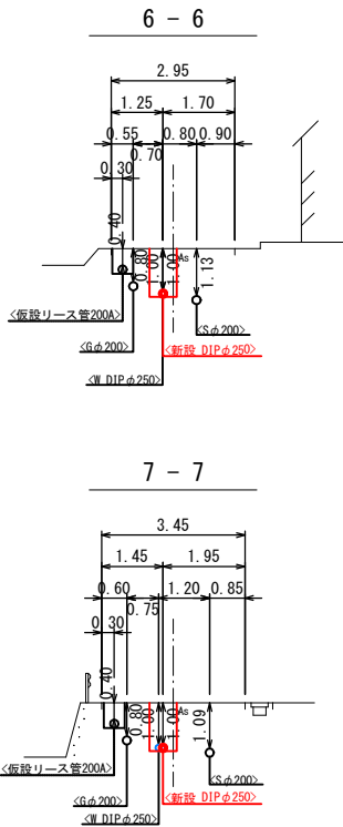
横断面図 S=1/100
