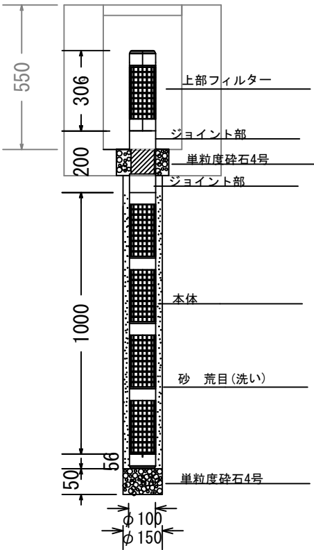
断面図
