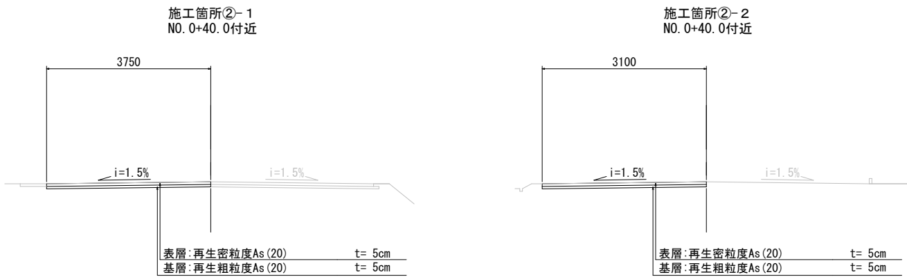
標準横断面図 S=1:50
