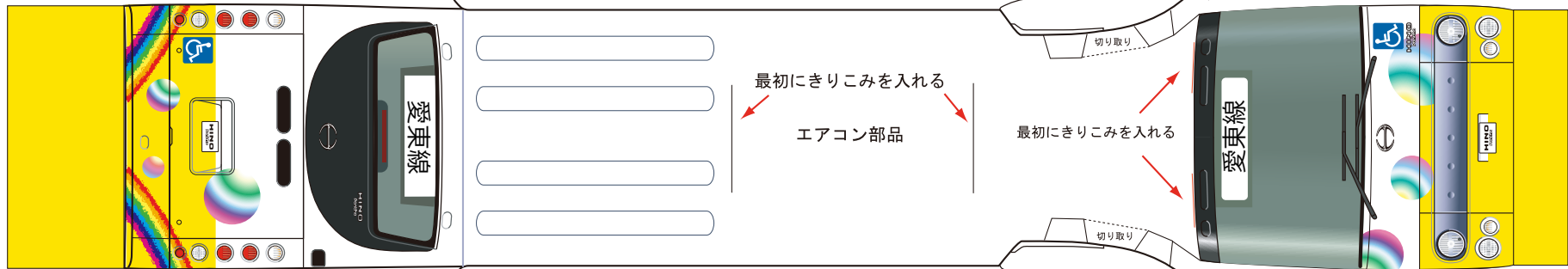
屋根部品
